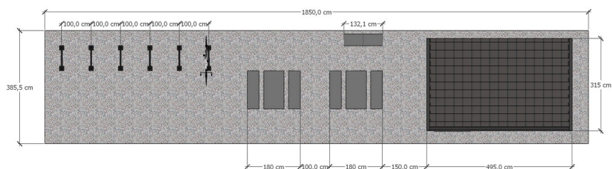
Ilustracja 30: Schemat wiaty w wariantcie 3.
